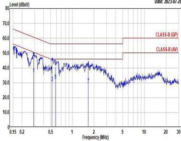
EMI: EN 55032 "B" (Conduction)
